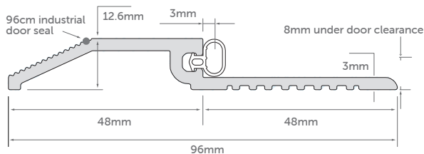
Mico Push Pad
