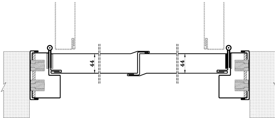
Double Door-set
